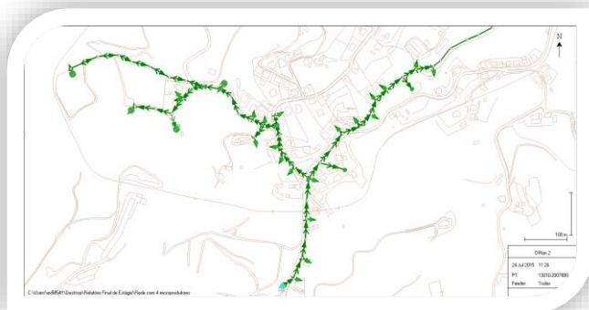
Rede com Requerente de 20,7 kVA e 4 Microprodutores
