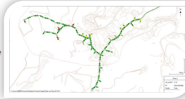
Rede com Requerente de 20,7 kVA
